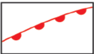
rim of active polje 浸食進行中のポリエ縁
