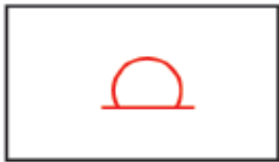
horizontal dry cave 乾いた横穴
