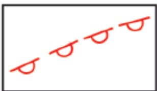
undefined rim of inactive polje ポリエ縁 (はっきりしない)
