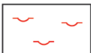
kamenitsas カメンティタ
