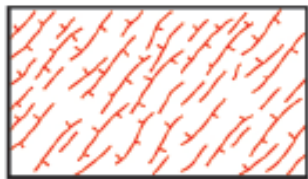
spitzkarren field 尖頂カレンフェルト
