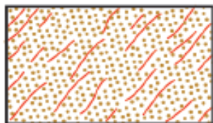
covered karren field 被覆カレンフェルト
