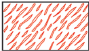
roundkarren field 円頂カレンフェルト
