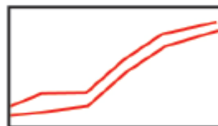
roofless cave 屋根なし洞窟
