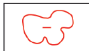
Uvala ウバラ(ドリーネが結合したもの)
