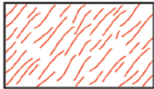
Karren field カレンフェルト
