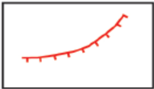
small scarp 小さい浸食による急斜面
