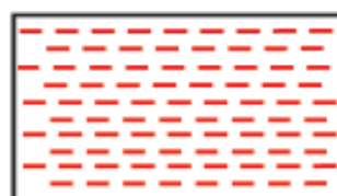
speleothems (not tufa) 鍾乳石
