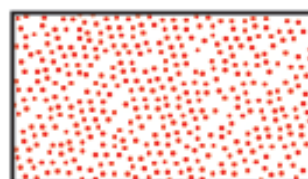
karstic infillings 石灰質の充填物
