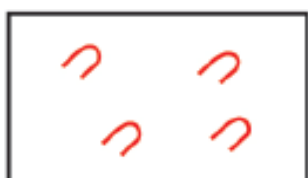
Heel-print karren Trittkarren 階段カッレン
