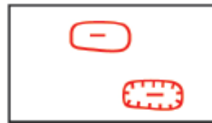
Doline doline with steep slopes ドリーネ(擂鉢状凹地、急斜面を伴う)
